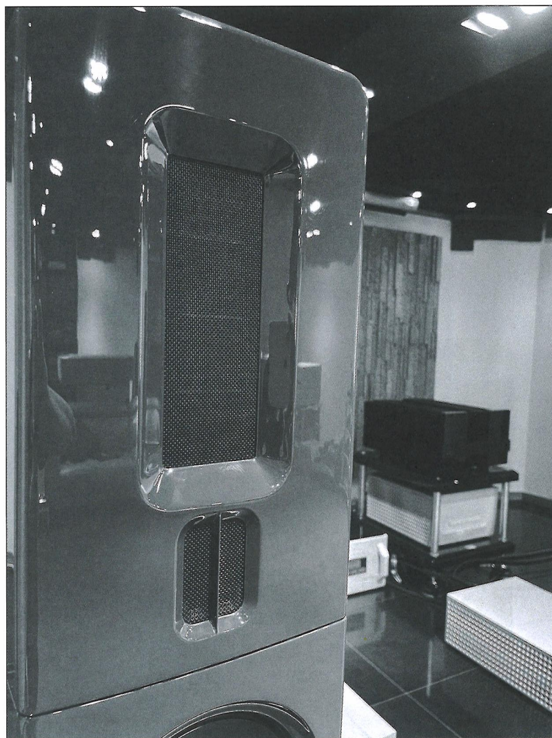
Aspen FR30 平面高音及平面中音單元，分別用上了 2.5 吋及 10 吋超低質量 Teonex 絲帶振膜。
