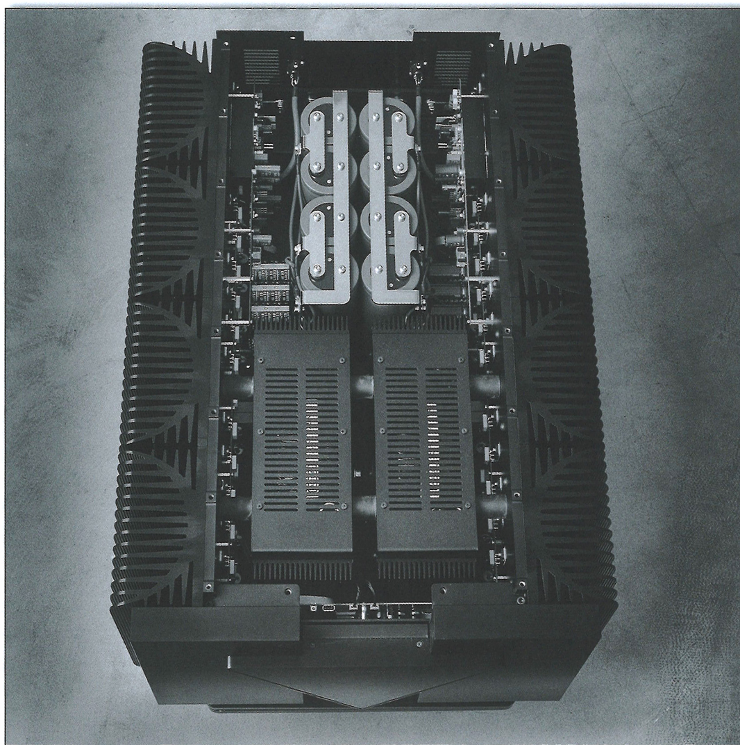
Apex 內部一覽。
