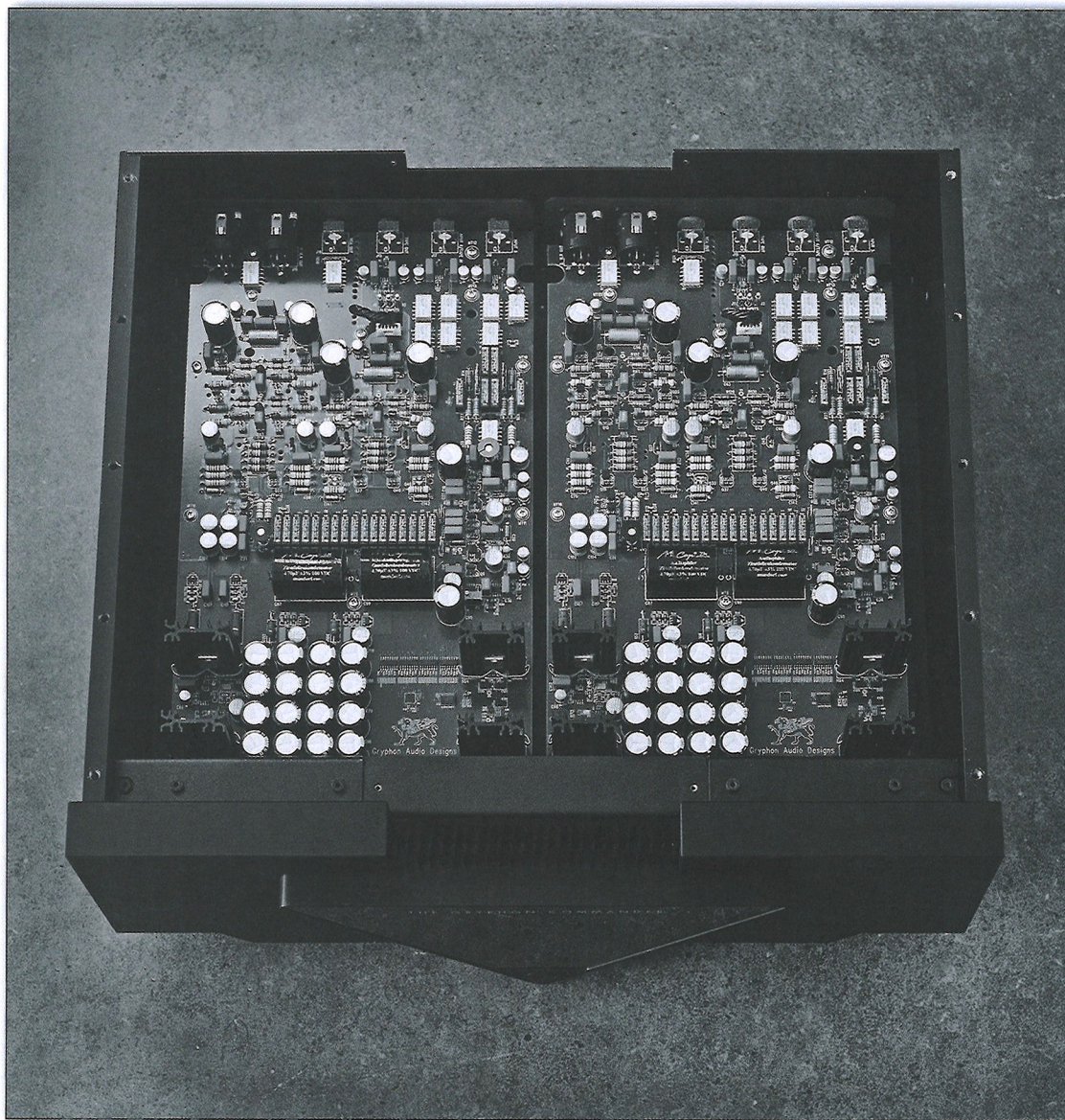
Commander 前級內部一覽。
